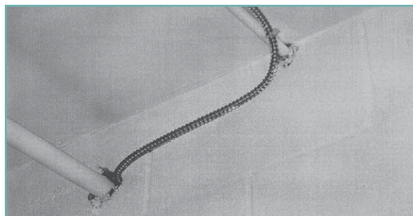
Figure 4-15 Points de pénétration de plomberie dans le mur d'un garage (photo : Proski Engineering Ltd.)
