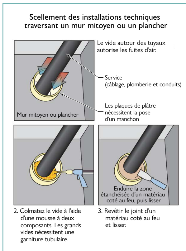
Figure 4-16 Calfeutrage des canalisations
