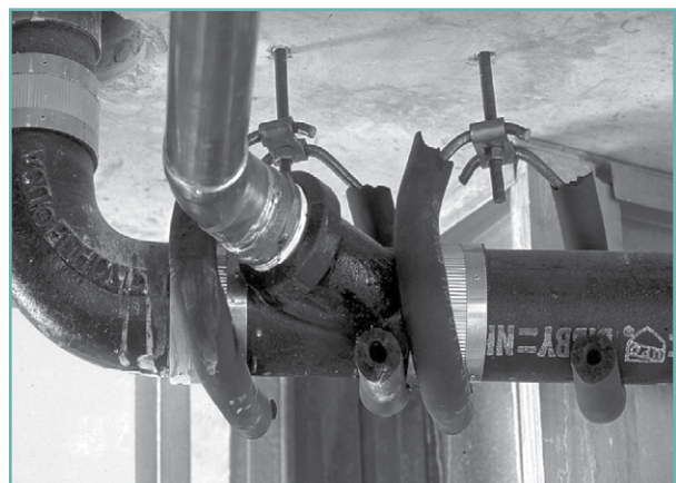
Figure 4-14 Points de pénétration de plomberie
