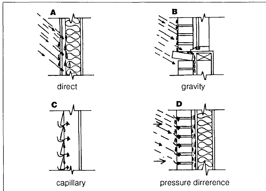
Fig. 27. Rain penetration
